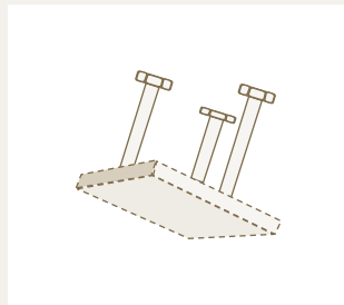
Abb. 1: Dübelleiste
